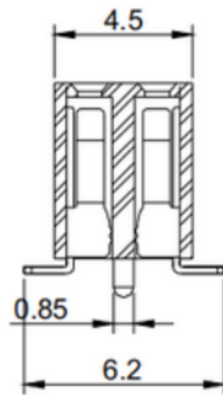
带定位柱
