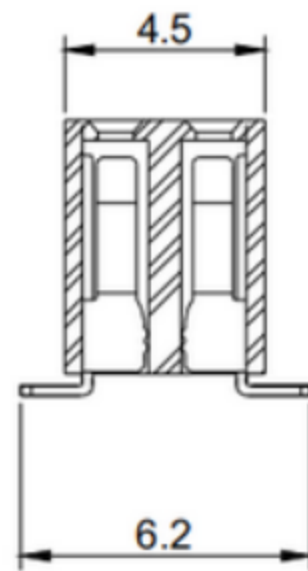
无定位柱
